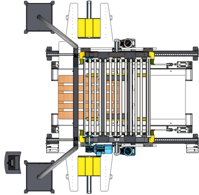
● Üst Görünüş ●
