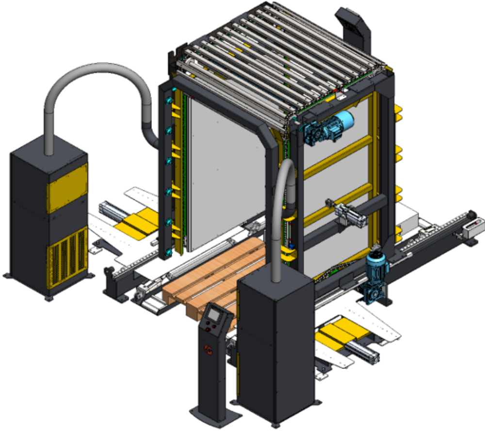
● Perspektif Görünüş ●
